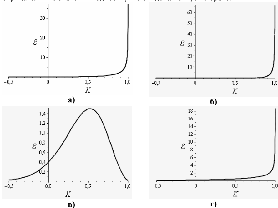
Рис 2. Примеры графиков плотности распределения годности размеров
