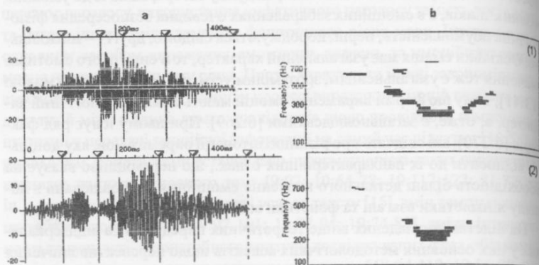
Рис. 1. Зміна інтенсивності (а) та спектрограма (б) звукового сигналу висловлювання "Come on" у першій ситуації (жіночий голос)
