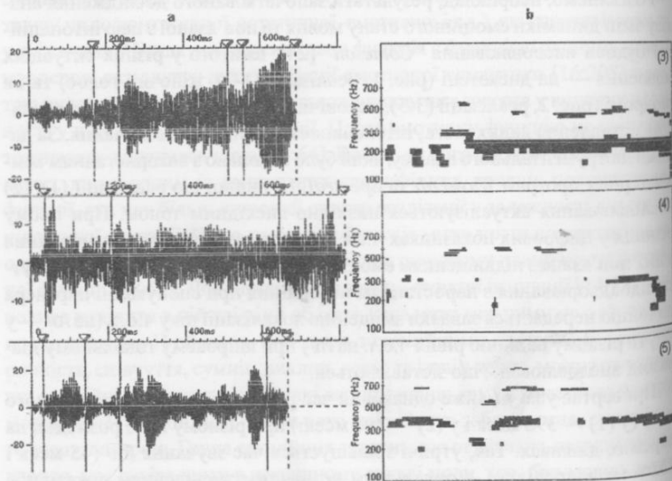
Рис. 2. Зміна інтенсивності (а) та спектрограма (б) звукового сигналу висловлювання "Come on" у другій ситуації (чоловічий голос)
