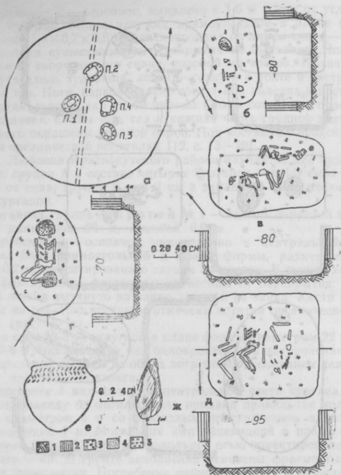
Рис. 2. План кургана № 1 и погребений из кургана у с. Любовка: 1 — материк, 2 — погребенная почва, 3 — материковый выкйд, 4 — охра, 5 — органическая подстилка
