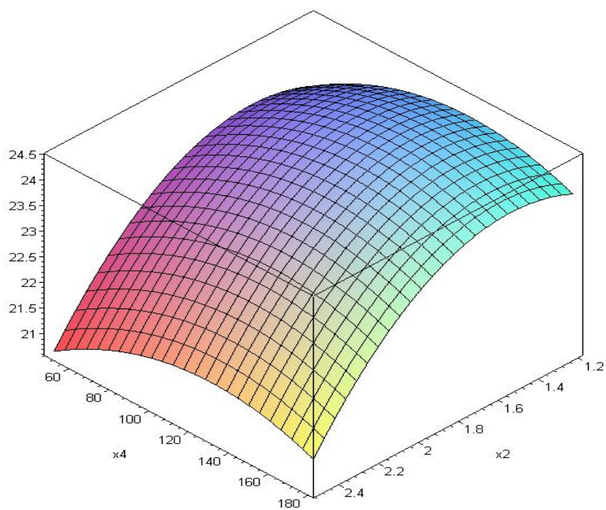
Рис. 3.8. Поверхня точності при знайденому оптимальному значенні подачі значення подачі x_1 = 0,94 мм., при оптимальній кількості обертань x_3 = 1410 об/хв.
