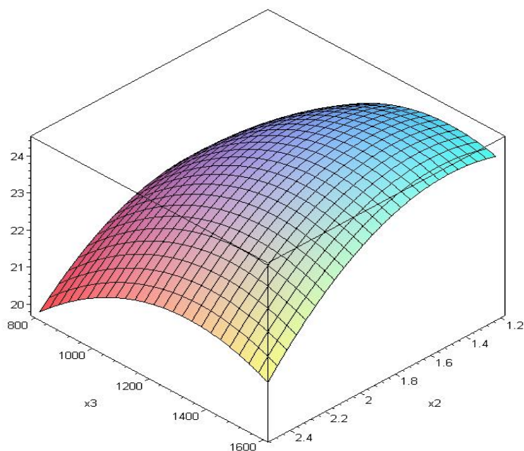
Рис. 3.7. Поверхня точності при знайденому значенні подачі x_1 = 0,94 мм., і з швидкістю різання x_4 = 128,31 м/с.
