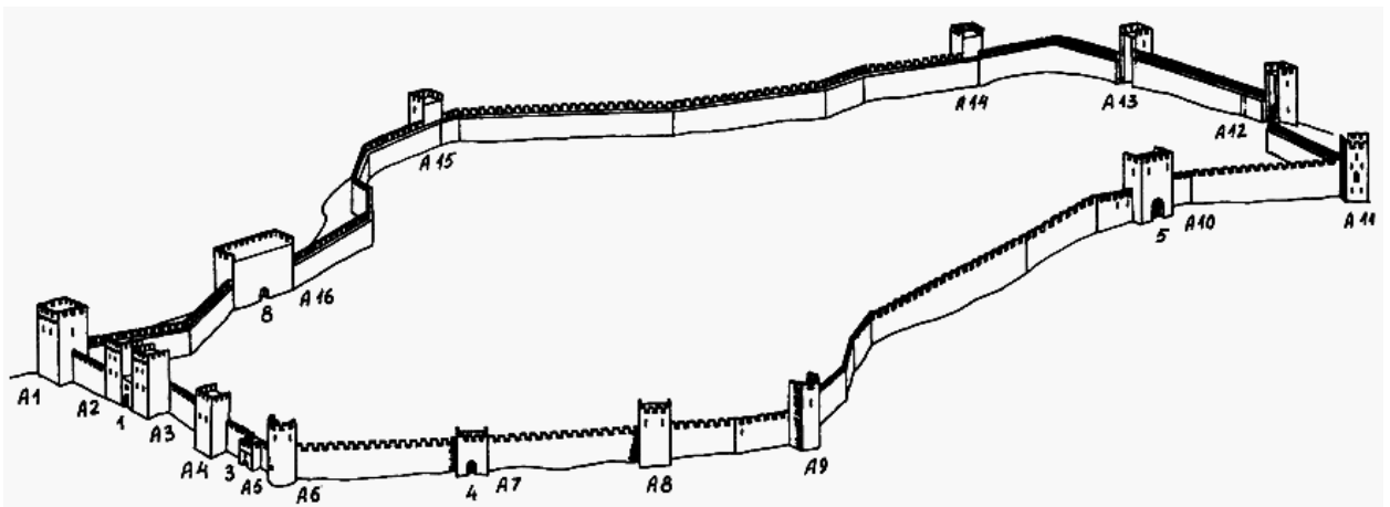
Мал. 6. Цитадель Кафи. Реконструкція (цифри без «А» – ворота; все інше – бапти)
