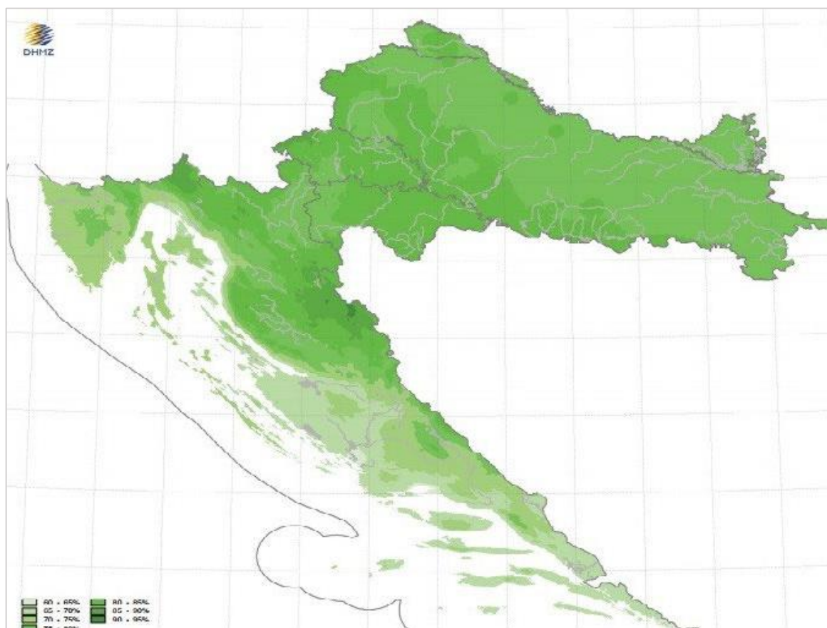
Рис. 2.10. Карта розподілу вологості по території Хорватії [12]
