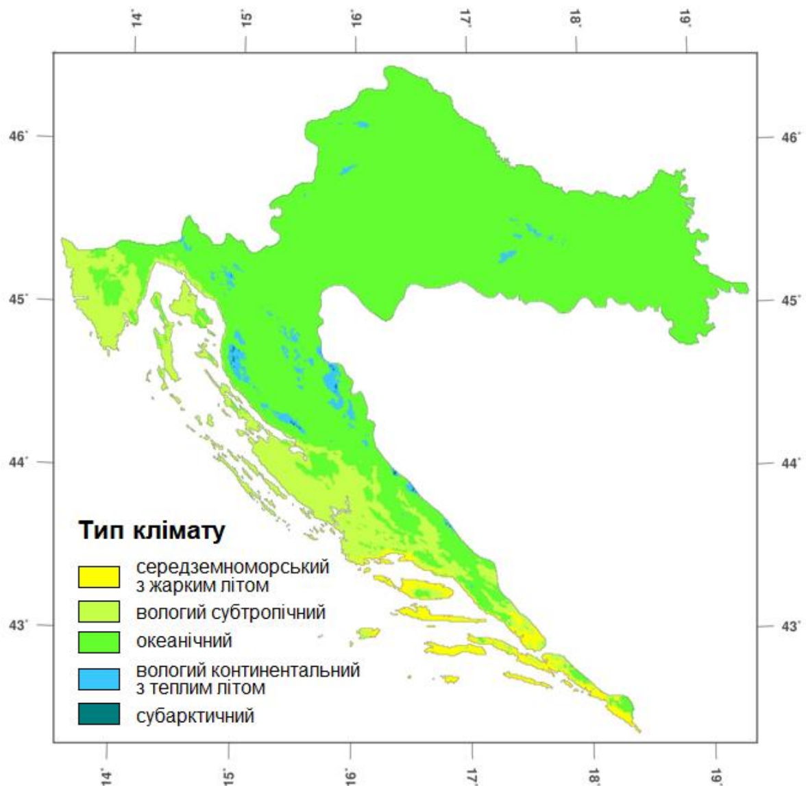
Рис. 2.8. Карта типів клімату Хорватії [1]
