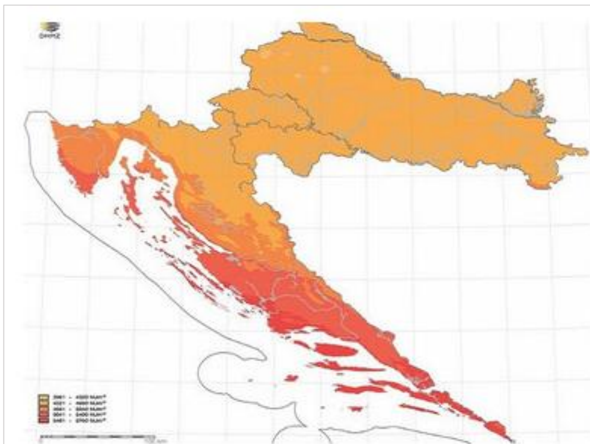
Рис. 2.9. Карта розподілу сонячної енергії по території Хорватії [12]
