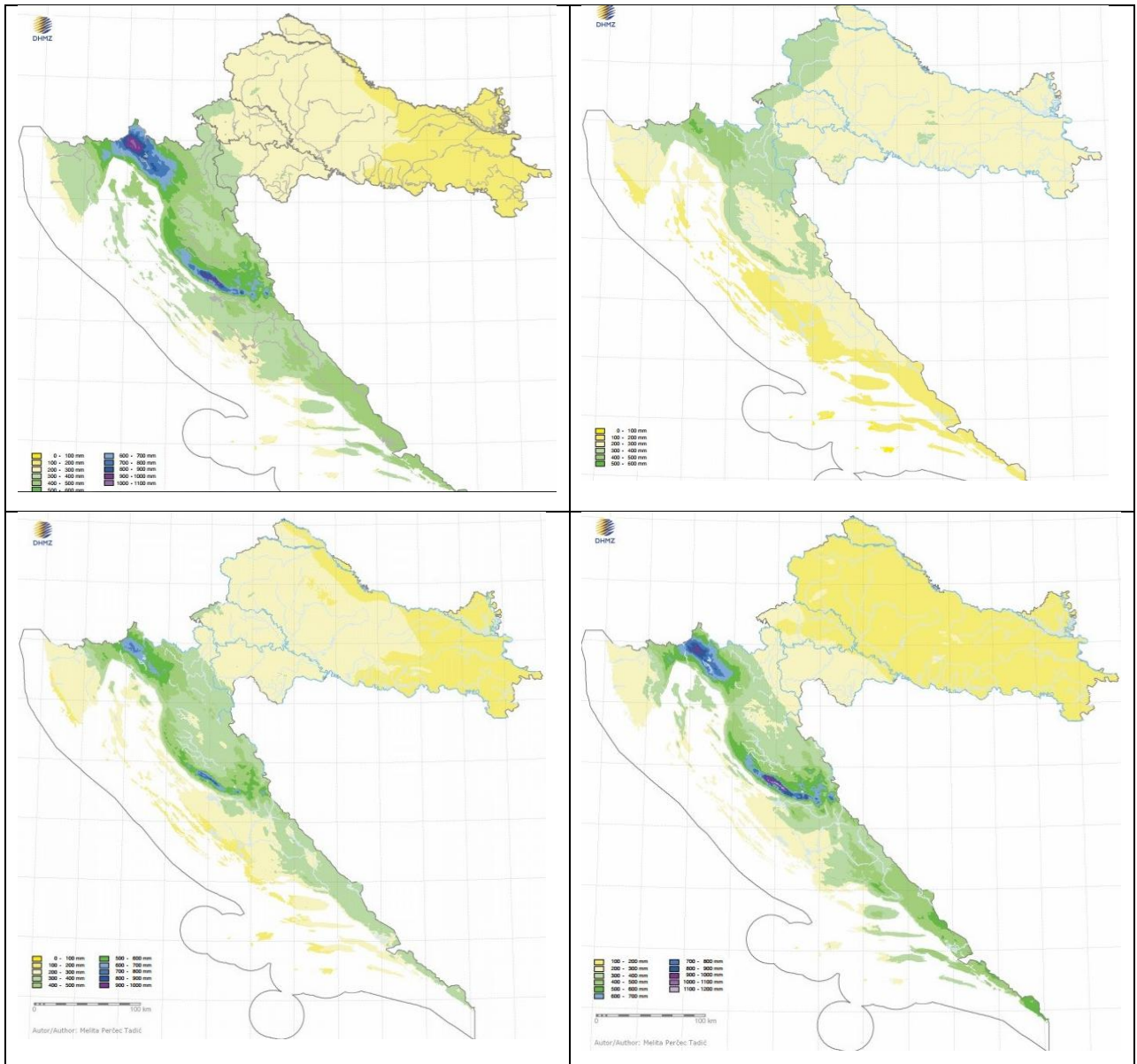
Рис. 2.11. Карти розподілу середньої кількості опадів за сезонами у Хорватії[12]
