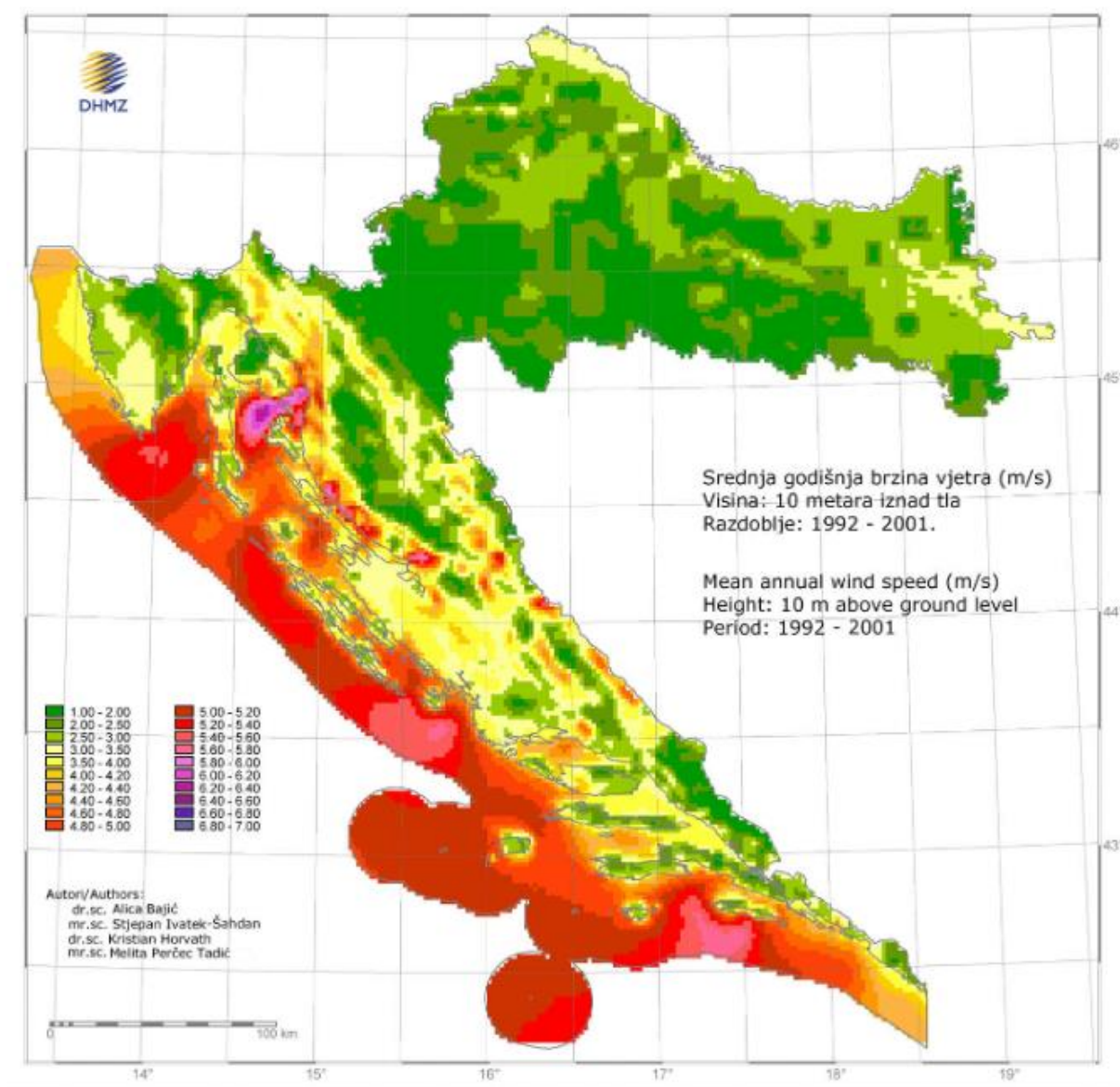
Рис. 2.8. Карта вітрів (швидкість) Хорватії [12]
