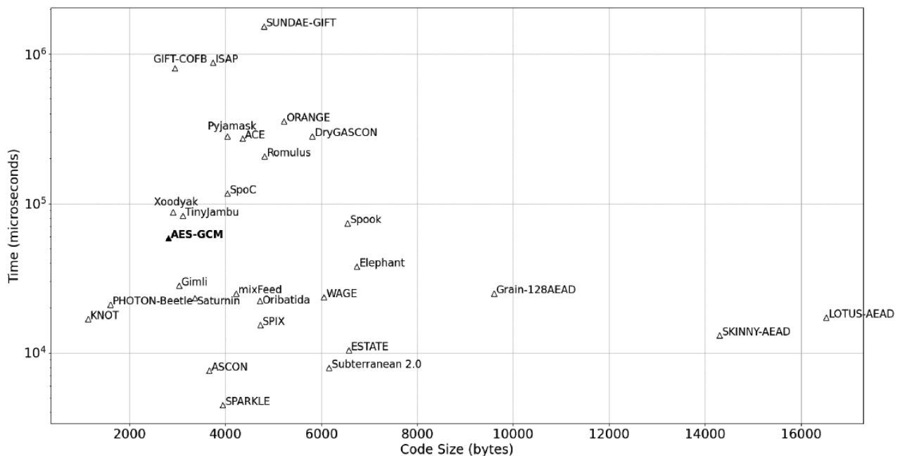
Рисунок 3 – Ефективність легковагових алгоритмів згідно NIST (Швидкість та розмір коду алгоритму)
