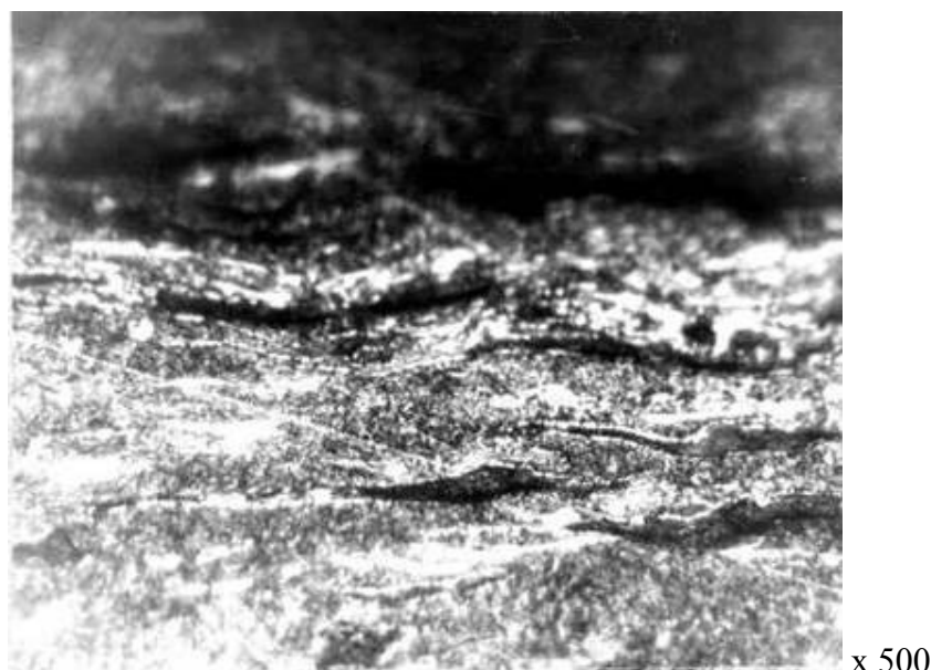
Рис. 3 – Текстурирование поверхностного слоя чугуна ВЧ60-2
