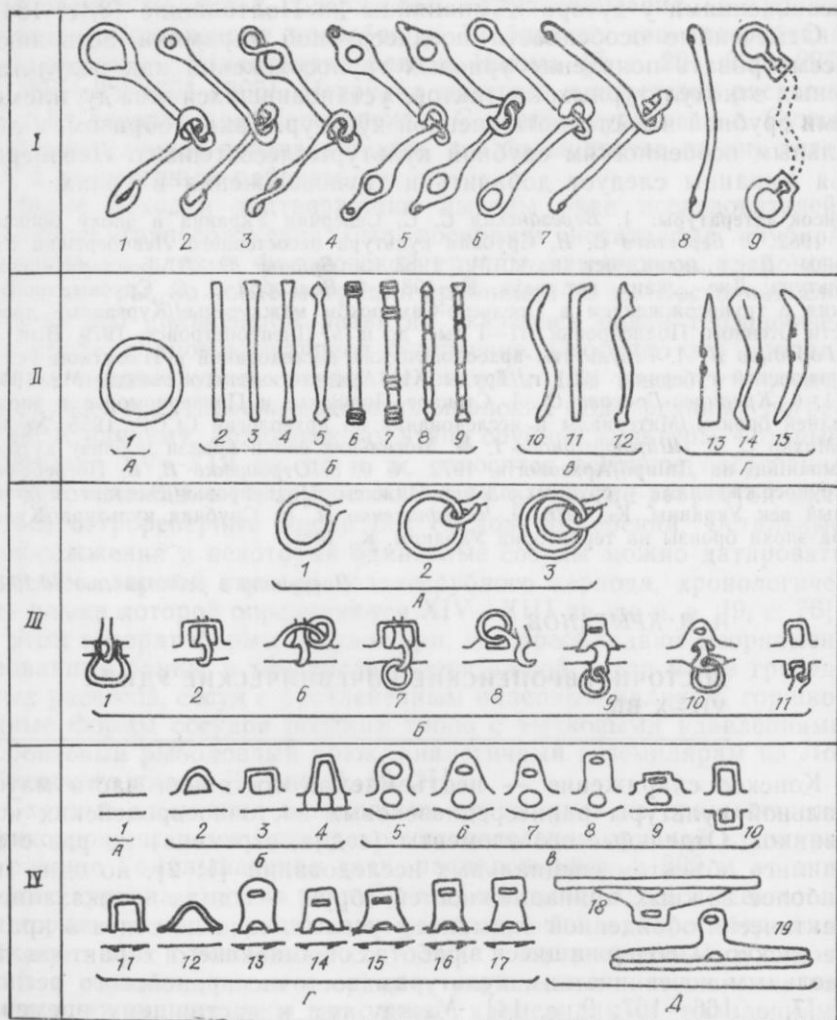
Рис. 1. Классификация отдельных элементов удил
