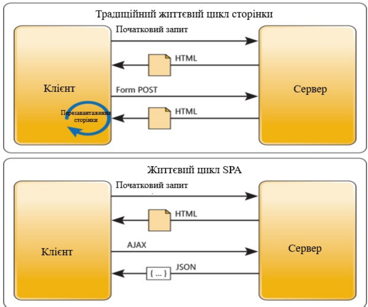
Рисунок 1.3 — Порівняння життєвого циклу традиційної сторінки та життєвого циклу SPA.
