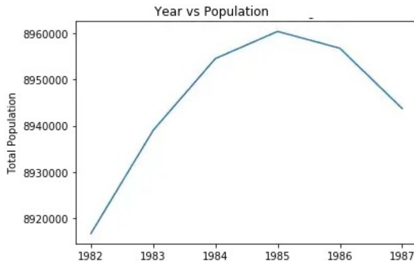
Рисунок 2.11 — Зображення побудованого простого лінійного графіку.
