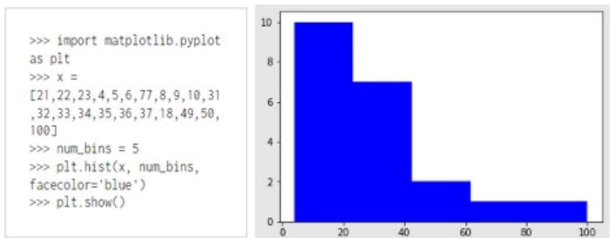
Рисунок 1.16 — Приклад 2: побудова гістограми.
