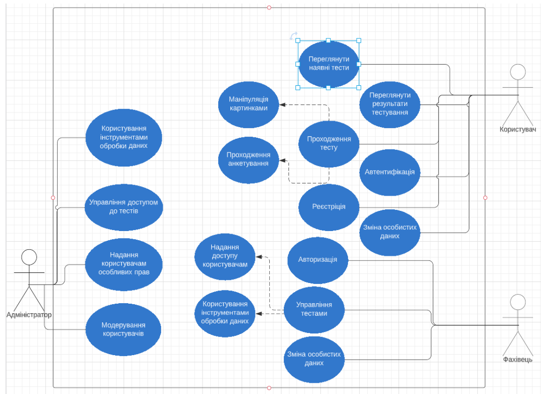
Рисунок 2.1 — Діаграма варіантів використання (UseCase diagram) “Комп’ютерної модель обробки великих обсягів даних”.
