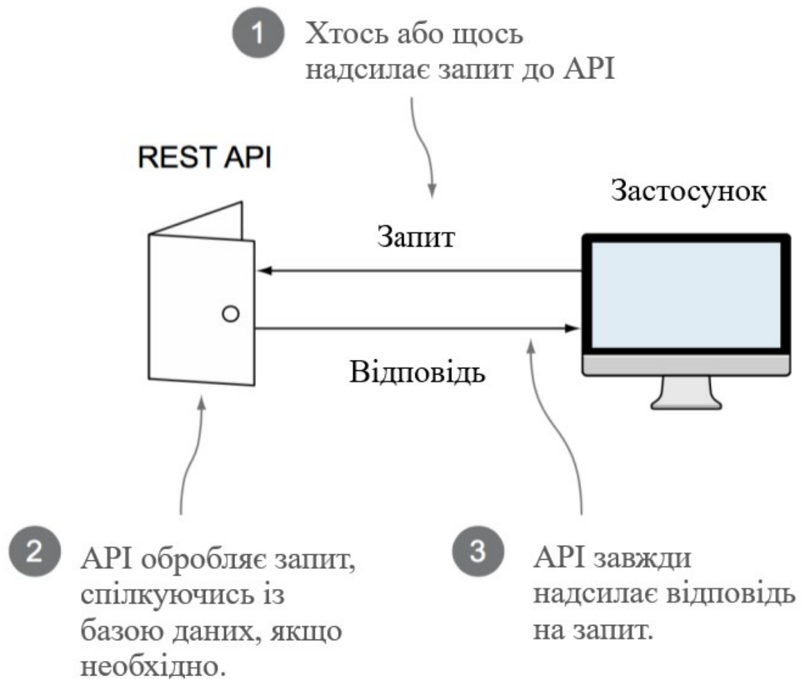
Рисунок 1.2 — Логіка REST API.
