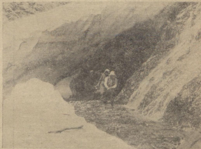
Вивчення льодовикових відкладів у верхів'ї ріки Кубані (Північний Кавказ).
