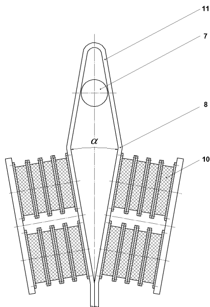
Рис. 2 – Гаситель коливань
