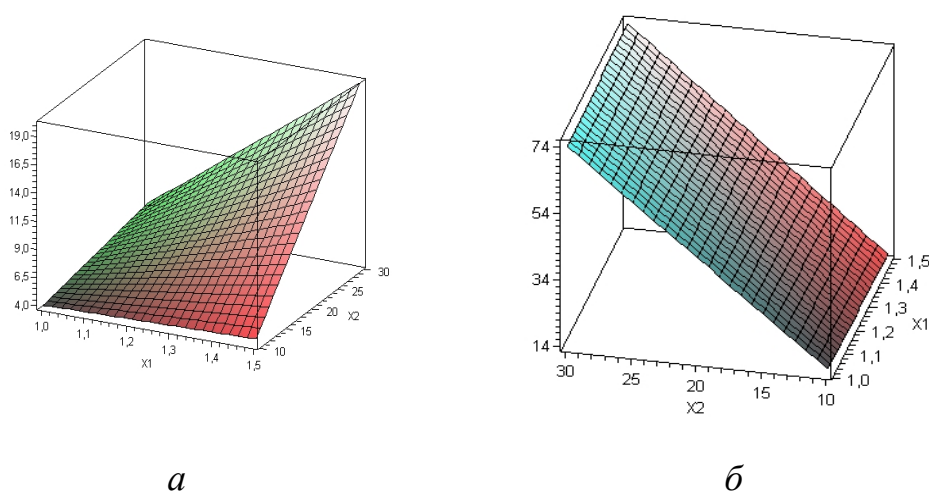
Рис. 2 – Поверхность микротвердости H(i, I_k/I_a) – (а) и толщины упрочненного слоя h(i, I_k/I_a) – (б) алюминиевого сплава Д16
