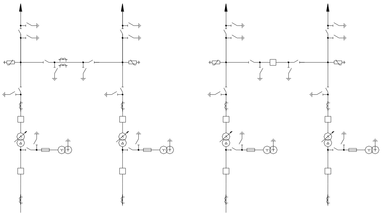
Рис. 1.5. Варіанти схем РПВН підстанцій споживачів
