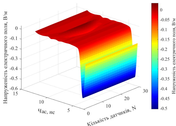
Рис. 3.30. Часові залежності електромагнітного поля для випадку зсуву часового вікна ліворуч від початкової позиції
