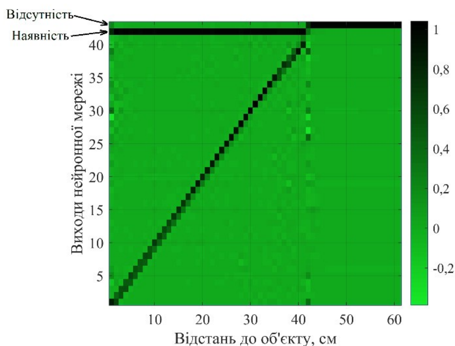
Рис 3.3. Значення вихідних нейронів ШНМ зі структурою 769-2000-1000-200-100-43 для різних відстаней до прихованого об'єкту при його поздовжньому зміщенні на 4 мм без використання SoftMax
