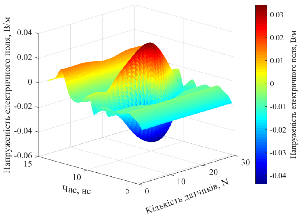
Рис. 3.32. Часові залежності електромагнітного поля для випадку зсуву часового вікна праворуч від початкової позиції
