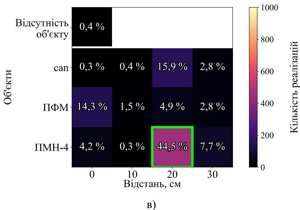
Рис. 4.30. Результат розпізнавання міни ПМН-4 на відстані 20 см для рівнів сигнал-шум: а) 25 дБ, б) 15 дБ, в) 5 дБ
