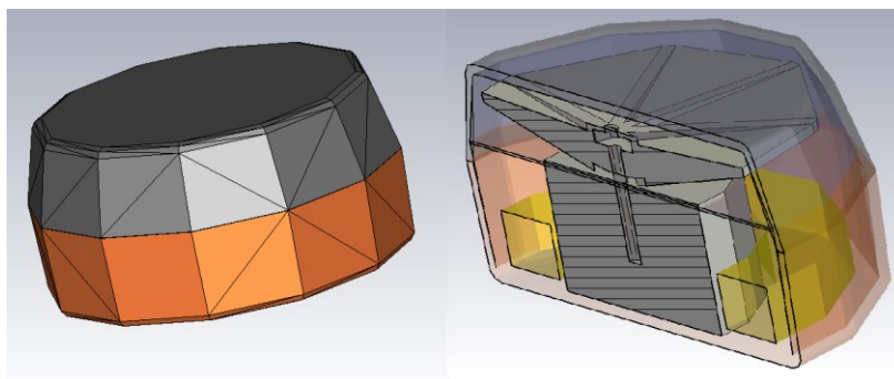
Рис. 4.5. Зовнішній вигляд моделі міни ПМН-4
