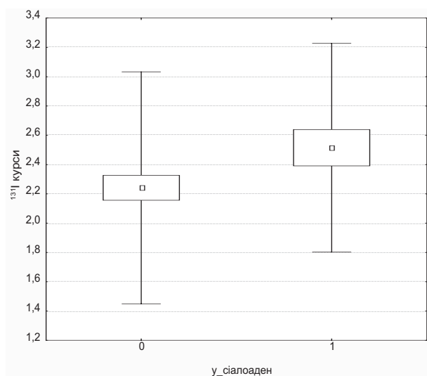
Рис. 3. Коробчасті графіки кількості курсів ^{131}\text{I} (зліва) та загальною активністю РНТ (справа) у хворих на РЩЗ з огляду на появу (1) та неяви (0) сіалоаденіту після лікування
