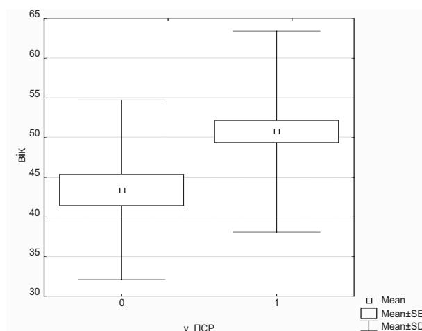
Рис. 5. Коробчасті графіки віку хворих на РЩЗ з огляду на появу (1) та неяви (0) порушення серцевого ритму після лікування
