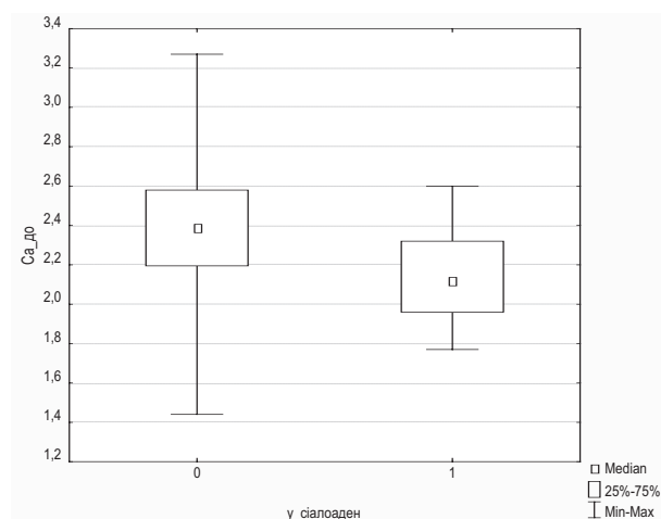
Рис. 4. Коробчасті графіки рівня Са у крові хворих на РЩЗ до проведення спеціального лікування з огляду на появу (1) та неяви (0) сіалоаденіту після лікування
