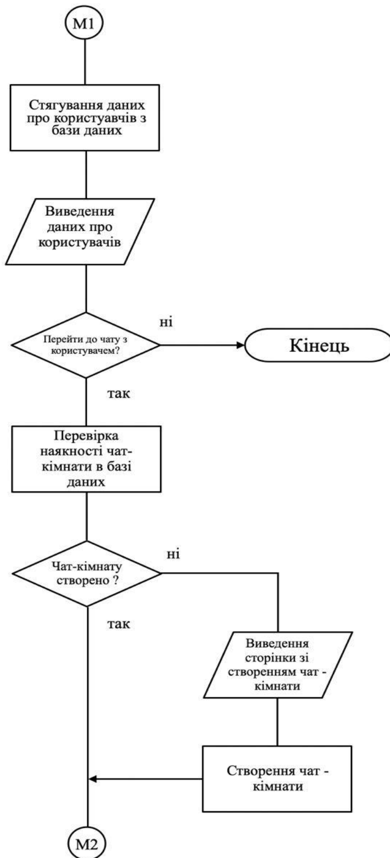
Рисунок 4.5 – Частина блок-схеми основної програми – бізнес-логіка на головній сторінці та сторінці створення чату
