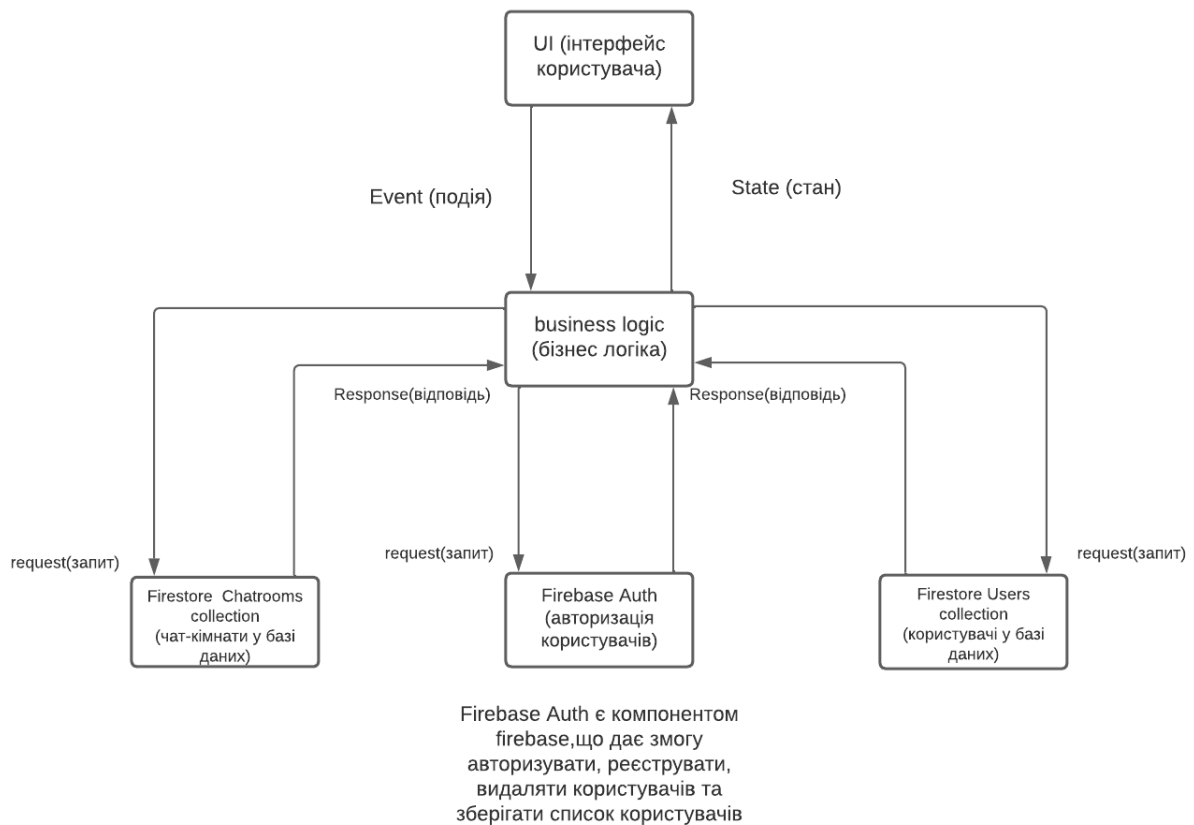
Рисунок 3.4 – Функціональна схема архітектури представлення BLoC (Business Logic of Component)
