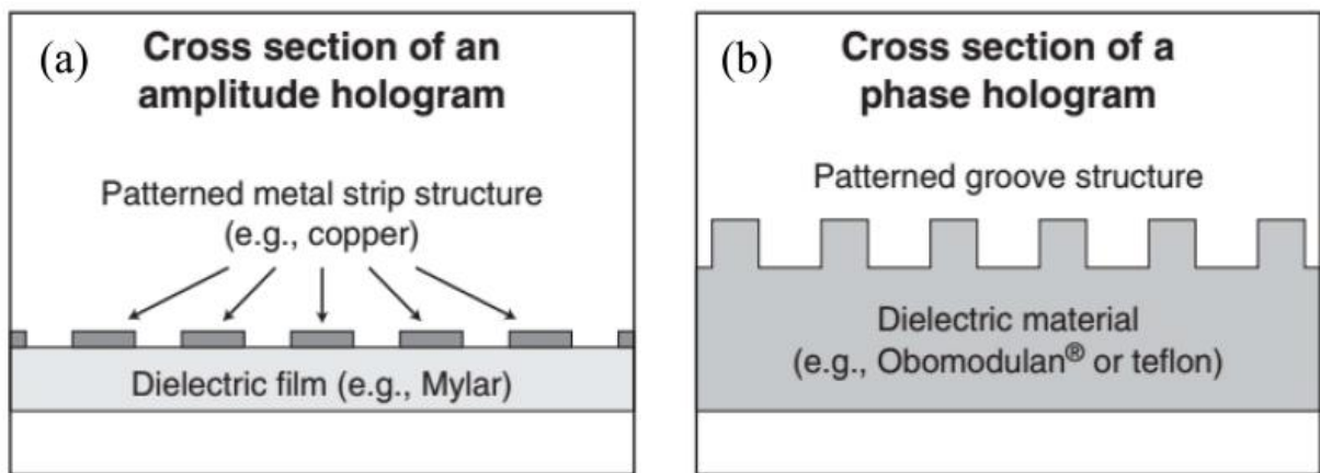
Рис. 1.6. Локальні решітчасті структури. а) амплітудні голограми; (б) фазові голограми
