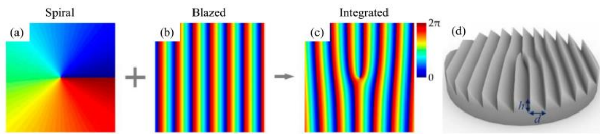
Рис. 1.5. Фазовий розподіл та ідея тривимірної схематичної структури ТГц РК роздвоєної поляризаційної решітки. (a) Звичайний спіральний розподіл фаз; (b) введено градієнтний розподіл фази; (c) інтегрований розподіл фаз; (d) ідеальна 3D РК роздвоєна поляризаційна решітка
