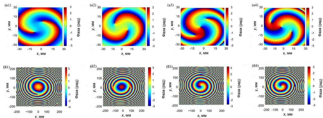
Рис. 2.6 Розрахункові поперечні розподіли фаз для E_x (перший, третій стовпець) та E_y (другий, четвертий стовпці) компонент поля лазерних пучків, що збуджуються модою TE_{01} , у зоні Френеля (a1 – a4) та в дальній (b1 – b4) зоні для n = 1 (перший та другий стовпці) і n = 2 (третій і четвертий стовпці)
