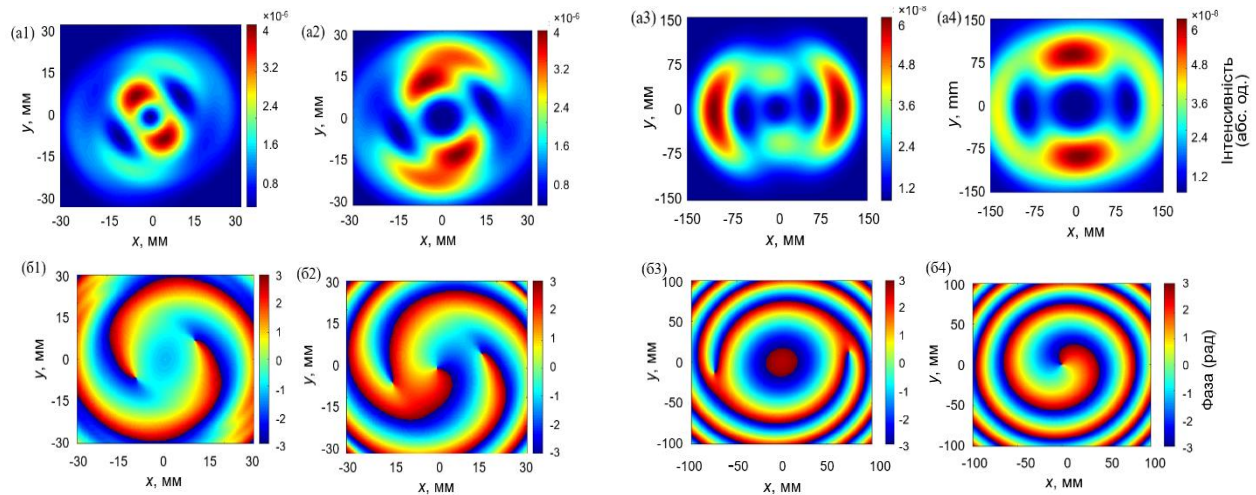
Рис. Б.3. Розрахункові поперечні розподіли інтенсивності (a1–a4) та фази (b1–b4) поля E_z компоненти лазерних пучків, збуджених модою TM_{01} , у зоні Френеля (перший та другий стовпець) та в дальній зоні (третій та четвертий стовпець). Перший і третій та другий і четвертий стовпці позначають n = 1 і n = 2 відповідно
