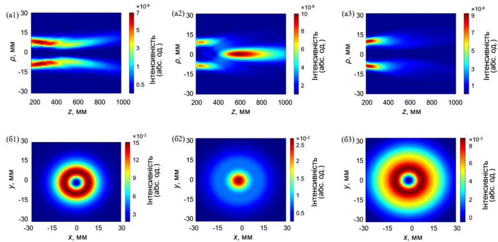
Рис 2.8 Розрахункові поздовжні (a1 – a3) та поперечні (b1 – b3) розподіли сумарних інтенсивностей поля лазерних пучків, що збуджуються модою TM_{01} , в зоні Френеля.
