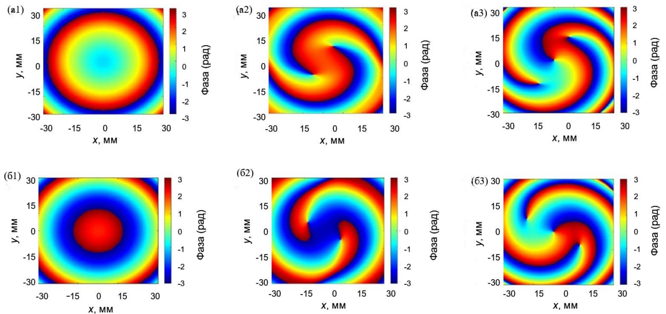
Рис. 2.21. Розрахункові поперечні розподіли фази поля для E_x (a1 – a3) та E_y (б1 – б3) компонент лазерних пучків, що збуджуються модою TE_{01} , в зоні Френеля для різних значень топологічного заряду. Перший, другий і третій стовпці позначають n = 0 , n = 1 і n = 2 відповідно
