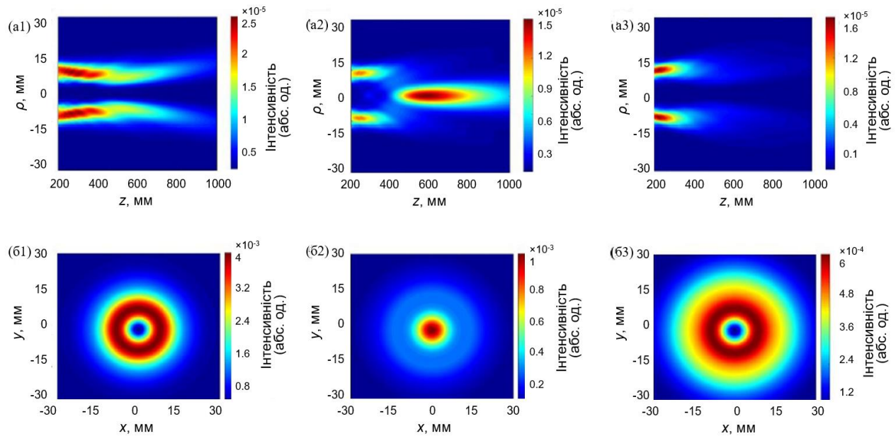
Рис 2.5 Розрахункові поздовжні (a1 – a3) та поперечні (b1 – b3) розподіли сумарних інтенсивностей поля лазерних пучків, що збуджуються модою TE_{01} , в зоні Френеля.
