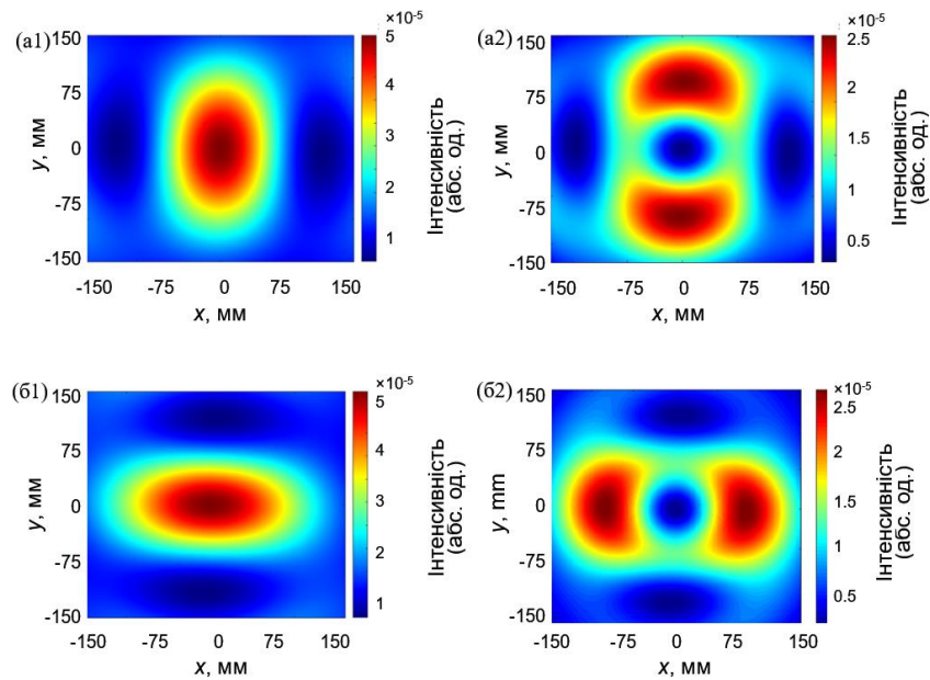
Рис. 2.27. Розрахункові поперечні розподіли інтенсивностей поля E_x (a1 – a2) та E_y (b1 – b2) компонентів лазерних пучків, що збуджуються модою TM_{01} , в дальній зоні для різних значень топологічного заряду. Перший та другий стовпці позначають n = 1 і n = 2 відповідно
