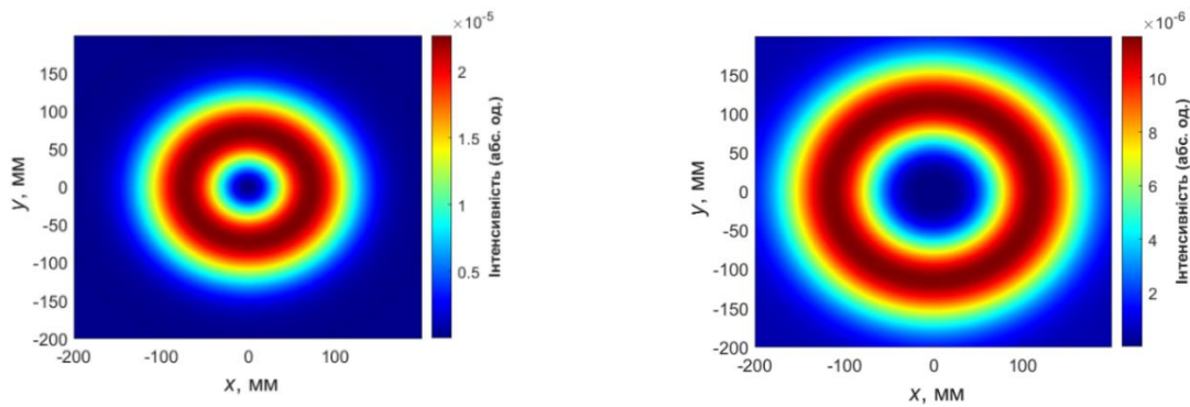
Рис 2.4 Розрахункові поперечні розподіли сумарної інтенсивності поля лазерних пучків, що збуджуються модою EH_{11} , в дальній зоні. Перший та другий стовпець позначають n = 1 і n = 2 відповідно
