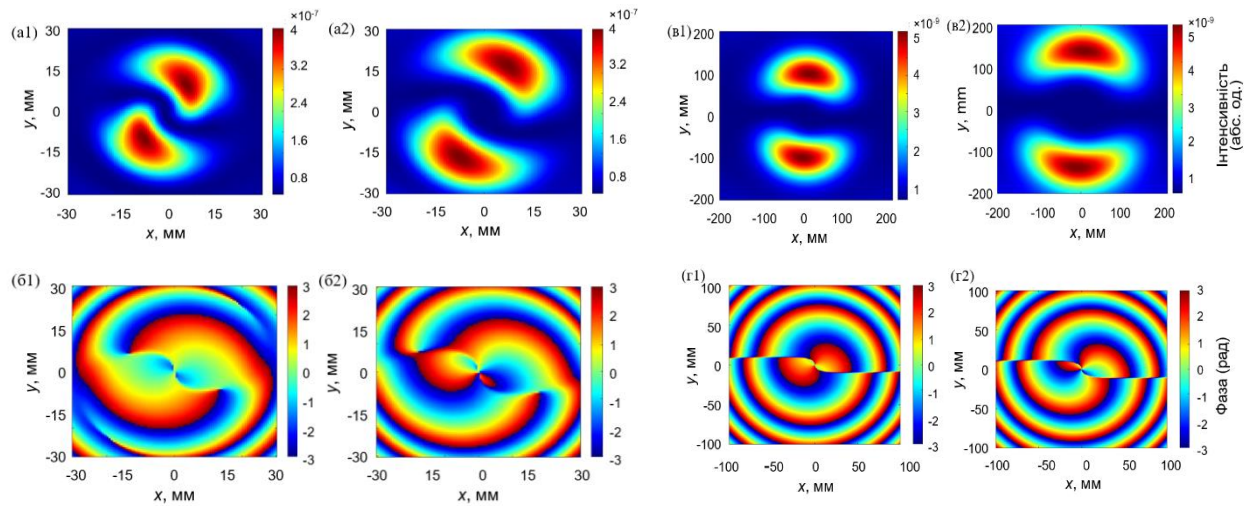
Рис. Б.1. Розрахункові поперечні розподіли інтенсивності (a1, a2, b1, b2) та фази (b1, b2, g1, g2) поля E_z компоненти лазерних пучків, збуджених модою EH_{11} , у зоні Френеля (а, б) та в дальній зоні (в, г). Перший і третій та другий і четвертий стовпці позначають n = 1 і n = 2 відповідно
