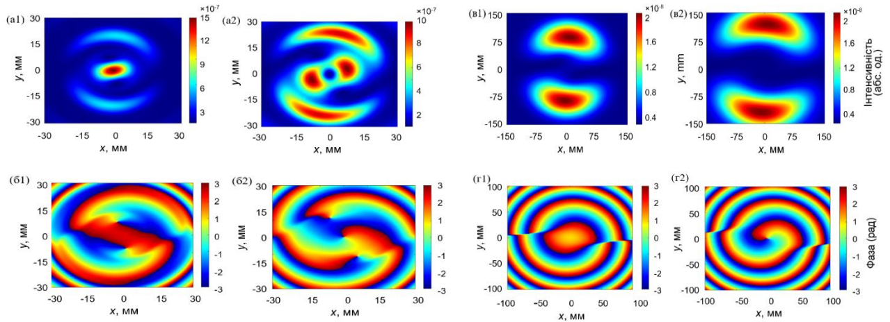
Рис. Б.4. Розрахункові поперечні розподіли інтенсивності (a1, a2, b1, b2) та фази (b1, b2, g1, g2) поля E_z компоненти лазерних пучків, збуджених модою TE_{11} , у зоні Френеля (рядки а, б) та в дальній зоні (рядки в, г). Перший і третій та другий і четвертий стовпці позначають n = 1 і n = 2 відповідно
