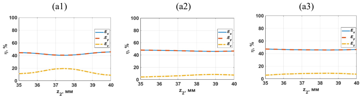
Рис. 3.16. Залежності відносного внеску потужності \eta компонент поля лазерних пучків, збуджених TM_{01} модою, в сумарну потужність у випадку гострого фокусування для топологічних зарядів n = 0 (a1), 1 (a2) і 2 (a3)
