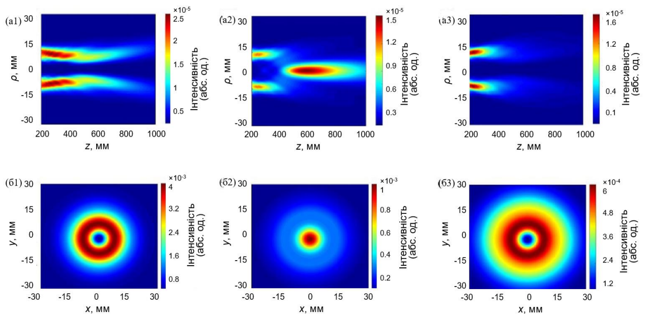
Рис. 2.20. Розрахункові повздовжні (a1–a3) та поперечні (б1 – б3) розподіли сумарної інтенсивності поля, збудженого модою TE_{01} , у зоні Френеля для різних значень топологічного заряду. Перший, другий і третій стовпці позначають n = 0 , n = 1 і n = 2 відповідно
