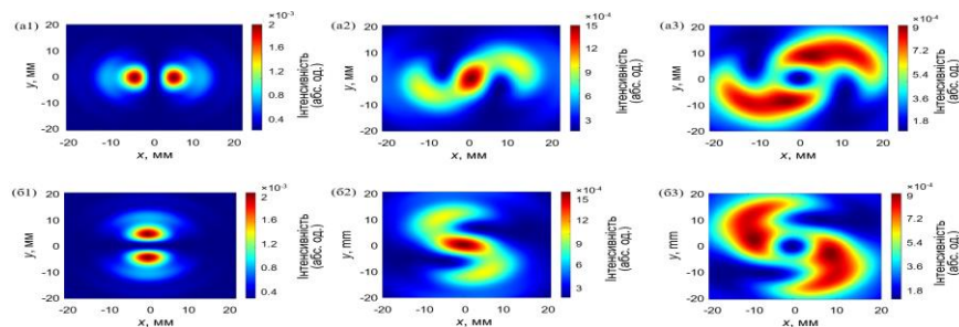
Рис. 2.9. Розрахункові поперечні розподіли інтенсивності поля E_x (a1 – a3) та E_y (b1 – b3) компонент лазерних пучків, збуджених модою TM_{01} , в зоні Френеля для різних значень топологічного заряду. Перший, другий і третій стовпці позначають
