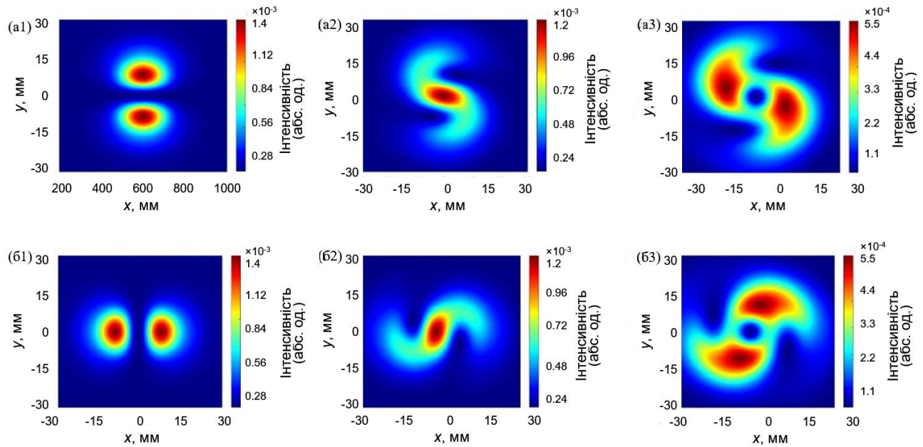
Рис. 2.21. Розрахункові поперечні розподіли інтенсивності поля E_x (a1 – a3) та E_y (б1 – б3) компонентів лазерних пучків, що збуджуються модою TE_{01} , у зоні Френеля для різних значень топологічного заряду. Перший, другий і третій стовпці позначають n = 0 , n = 1 і n = 2 відповідно
