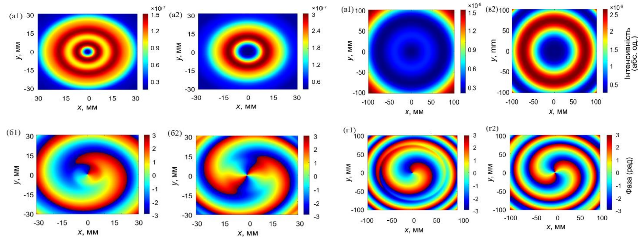
Рис. Б.2. Розрахункові поперечні розподіли інтенсивності (a1, a2, b1, b2) та фази (b1, b2, g1, g2) поля E_z компоненти лазерних пучків, збуджених модою TE_{01} , у зоні Френеля (рядки а, б) та в дальній зоні (рядки в, г). Перший і третій та другий і четвертий стовпці позначають n = 1 і n = 2 відповідно
