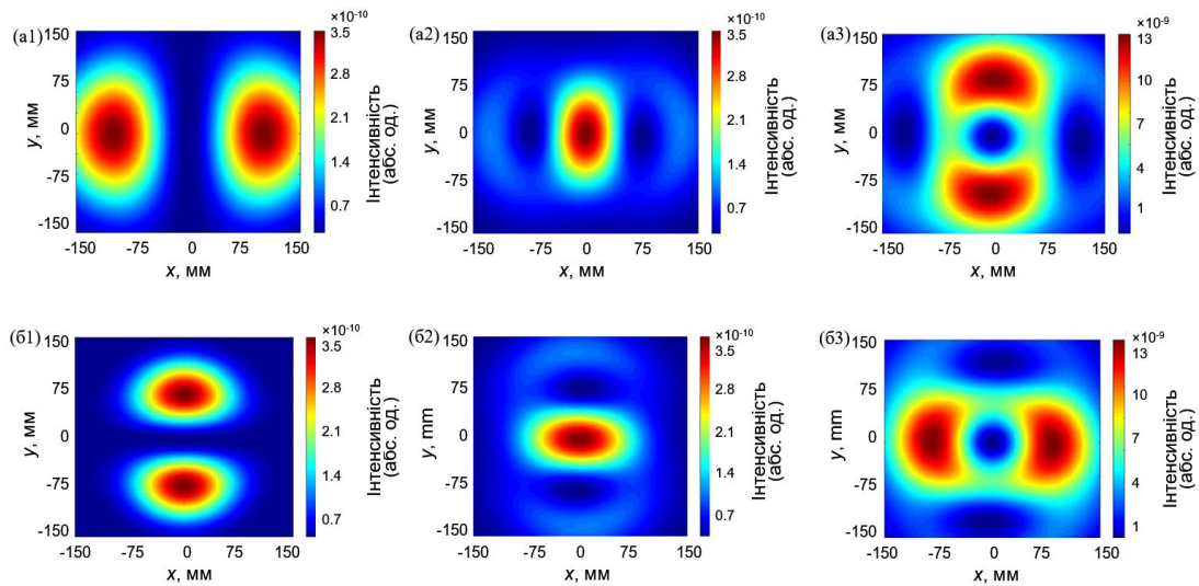
Рис. 2.11. Розрахункові поперечні розподіли інтенсивності поля E_x (a1 – a3) та E_y (b1 – b3) компонент лазерних пучків, збуджених модою TM_{01} , в дальній зоні для різних значень топологічного заряду. Перший, другий і третій стовпці позначають n = 0 , n = 1 і n = 2 відповідно
