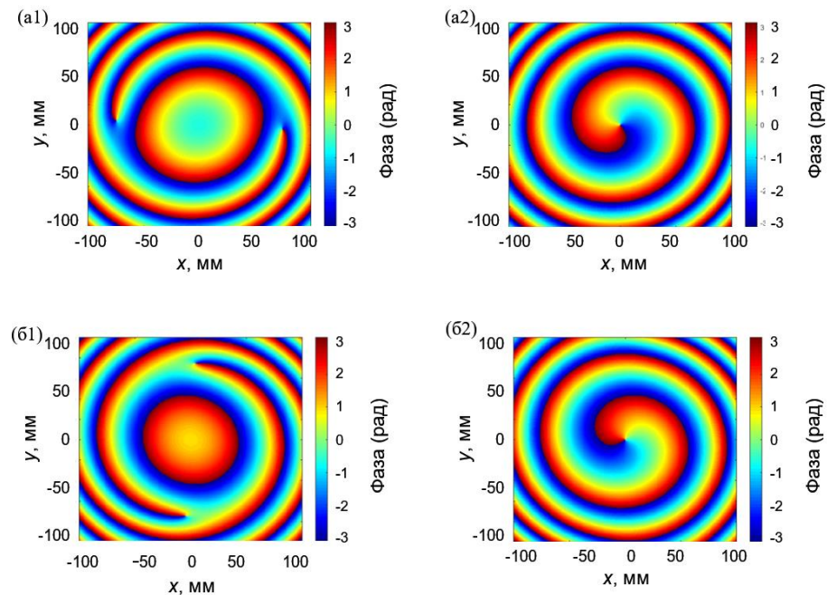
Рис. 2.12. Розрахункові поперечні розподіли фази поля для E_x (a1 – a2) та E_y (b1 – b2) компонент лазерних пучків, що збуджуються модою TM_{01} , у дальній зоні для різних значень топологічного заряду. Перший та другий стовпець відповідають n = 1 і n = 2 відповідно
