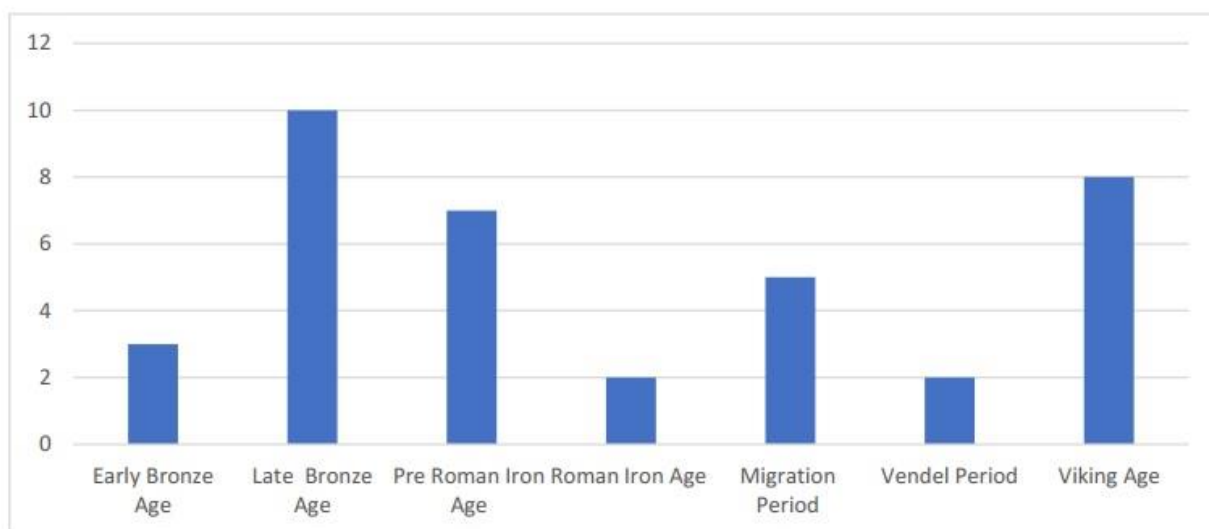
Діаграма 1. Радіовуглецеві дати кісткового матеріалу з болот в Упланді.
