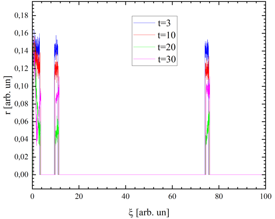
Рис. 2.11- Еволюція з часом радіусу однорідного згустку-передвісника (довжиною l_{pr} = \lambda/2 та густиною n_{pr} = n_b/2 , n_b – густина основного згустку) та двох віддалених головних однорідних згустків, довжина яких l_b = \lambda/4 . Радіус, струм та енергія згустків як і на рис. 2.7.
