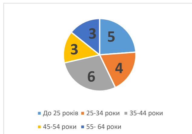
Рис. 3.2 Вік
