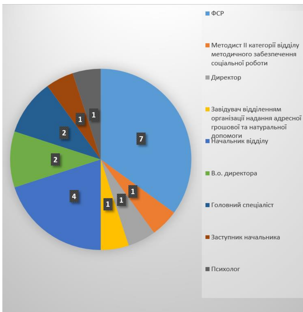
Рис. 3.4 Посада
