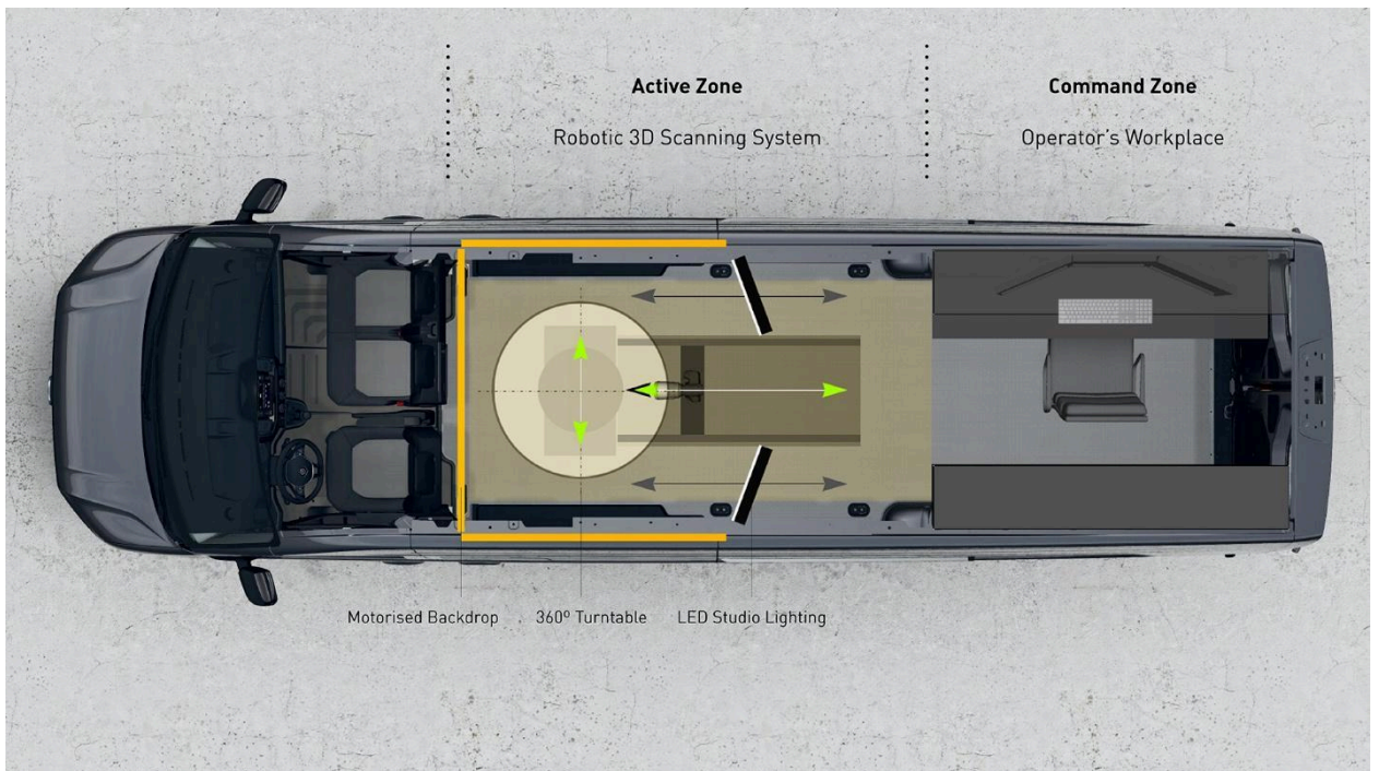
Рис. 2.3. ARK III - Мобільний блок оцифрування тривимірних об'єктів Джерело: [11]
