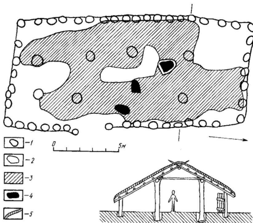
Рис. 1. Будешти. План та реконструкція будівлі 2. Умовні знаки: 1 – стовпові ями, 2 – інші ями, 3 – розвал обпаленої глиняної обмазки, 4 – вогнище, 5 – глиняна обмазка покрівалі.
